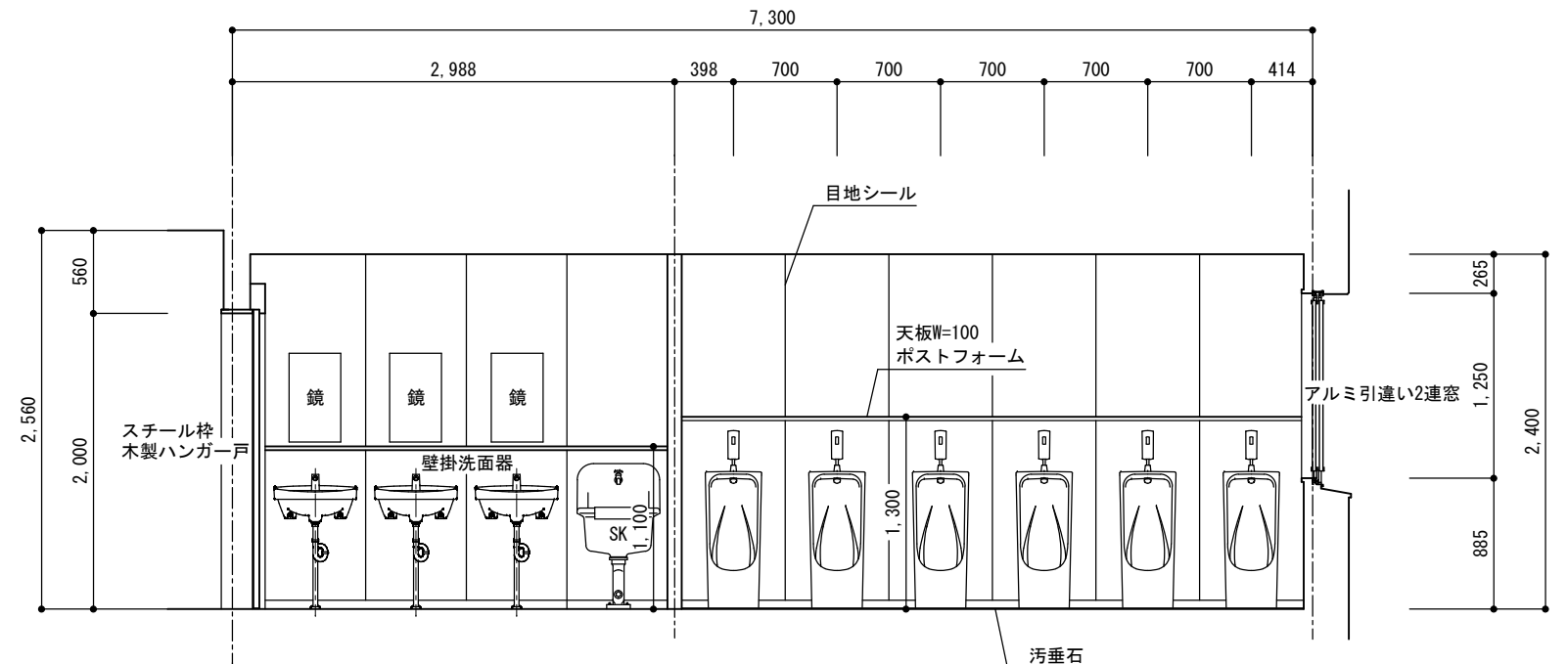
男子トイレ B面
