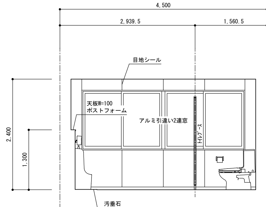
男子トイレ C面
