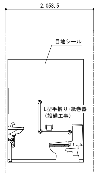
多目的トイレ C面
