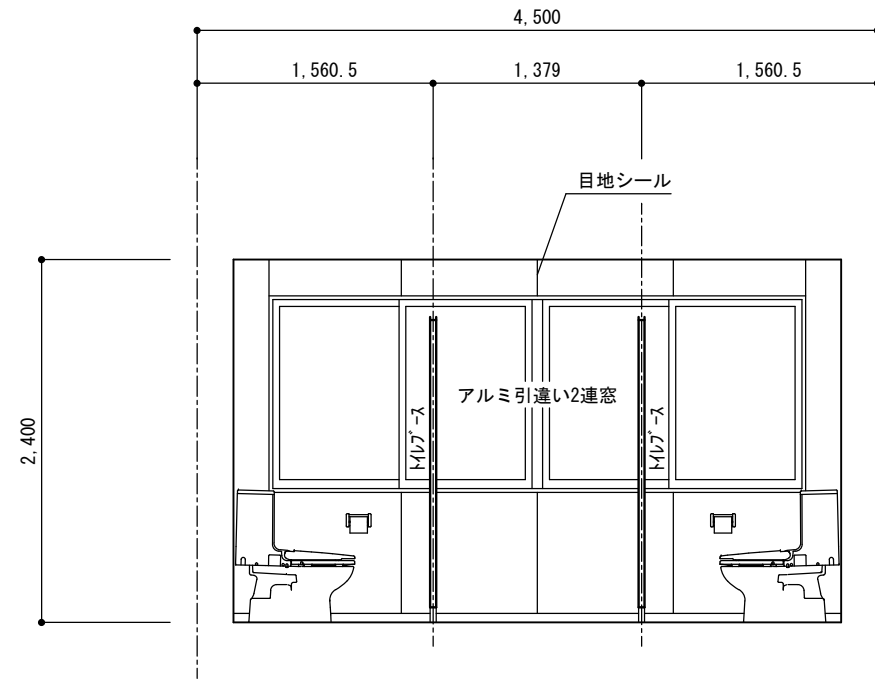
女子トイレ C面
