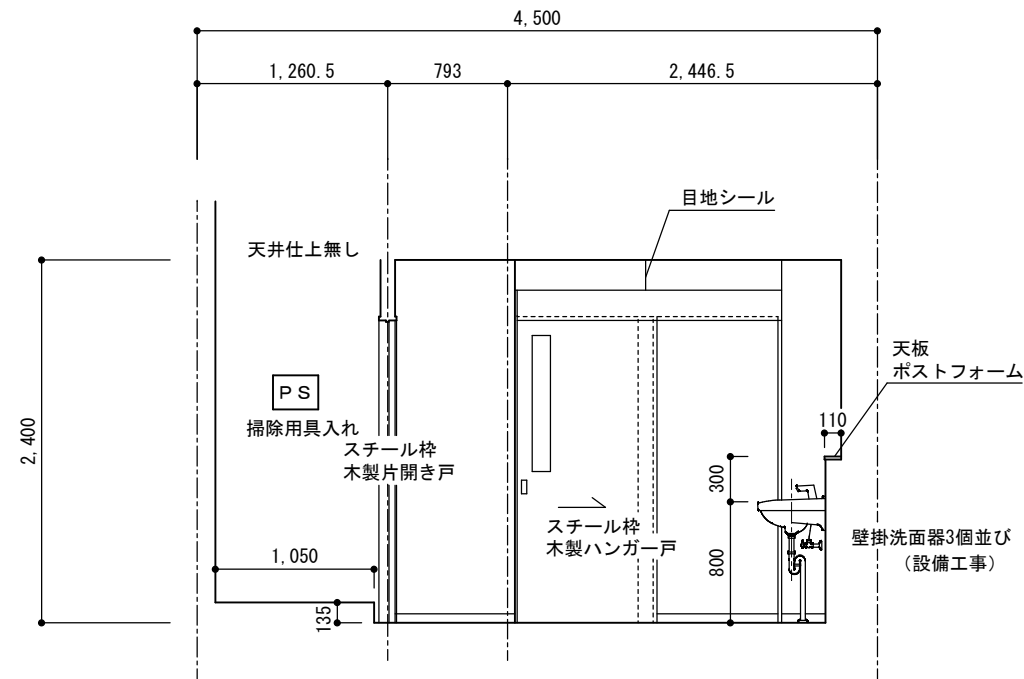
男子トイレ A面
