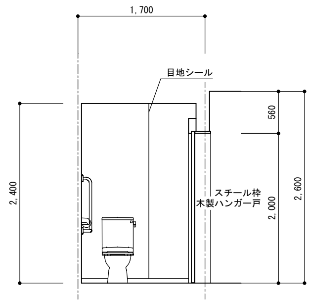
多目的トイレ D面
