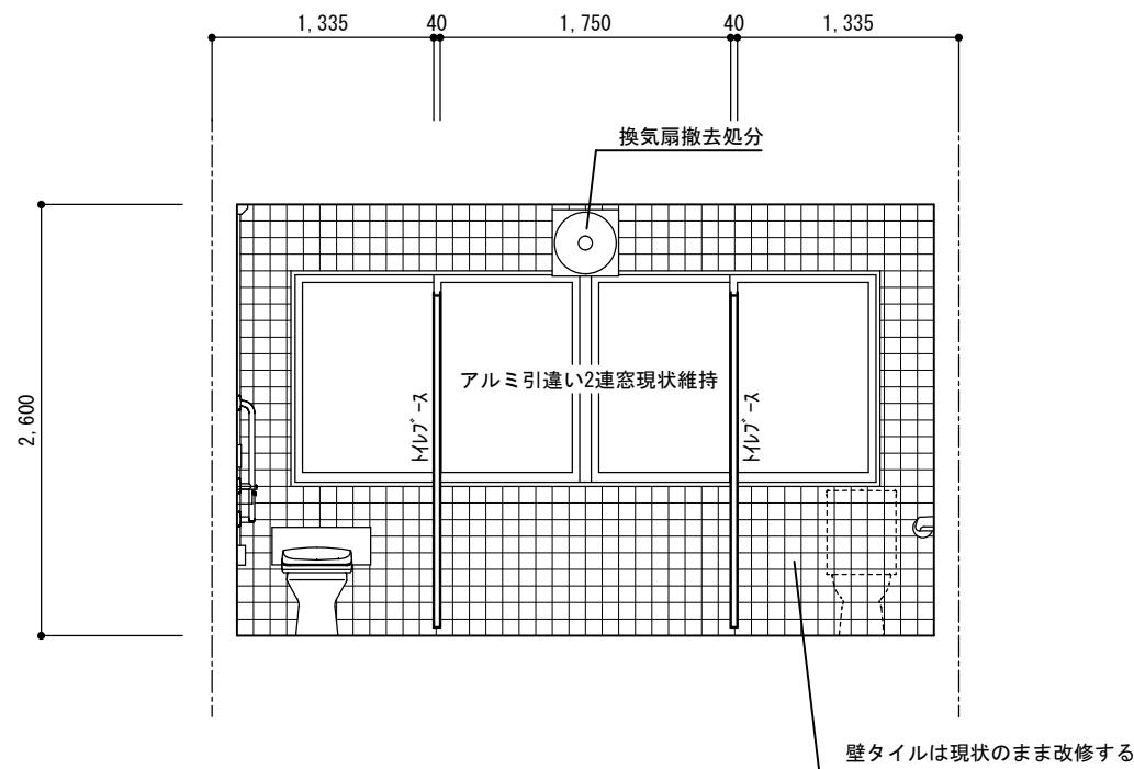
女子トイレ C面
