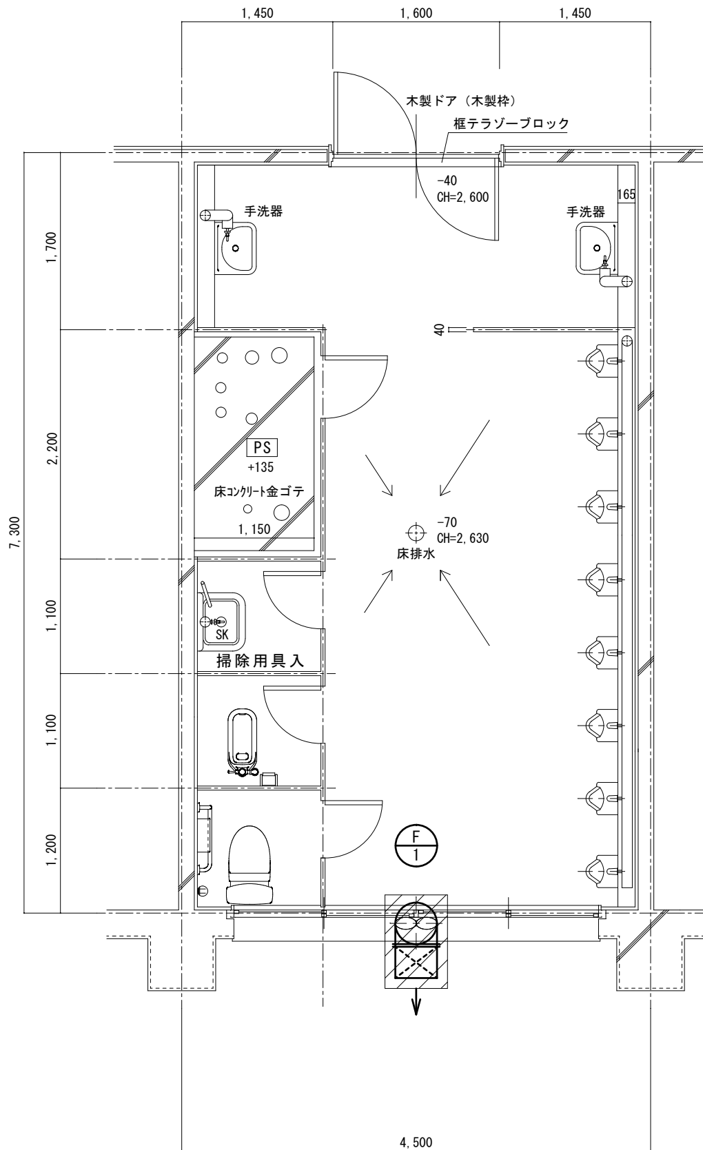
既存2階平面詳細図
