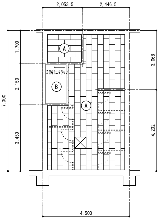
1. 3階天井伏図 1/100
