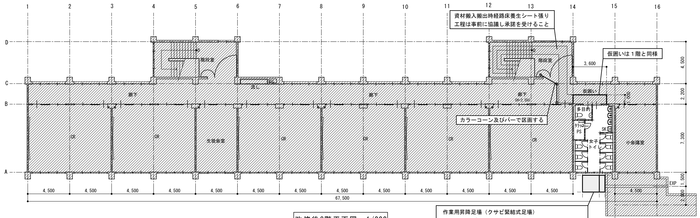
改修後3階平面図 1/200
