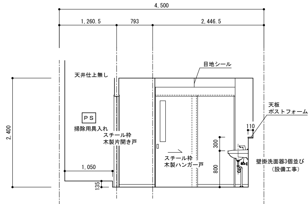
女子トイレ A面
