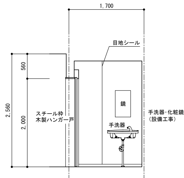
多目的トイレ B面
