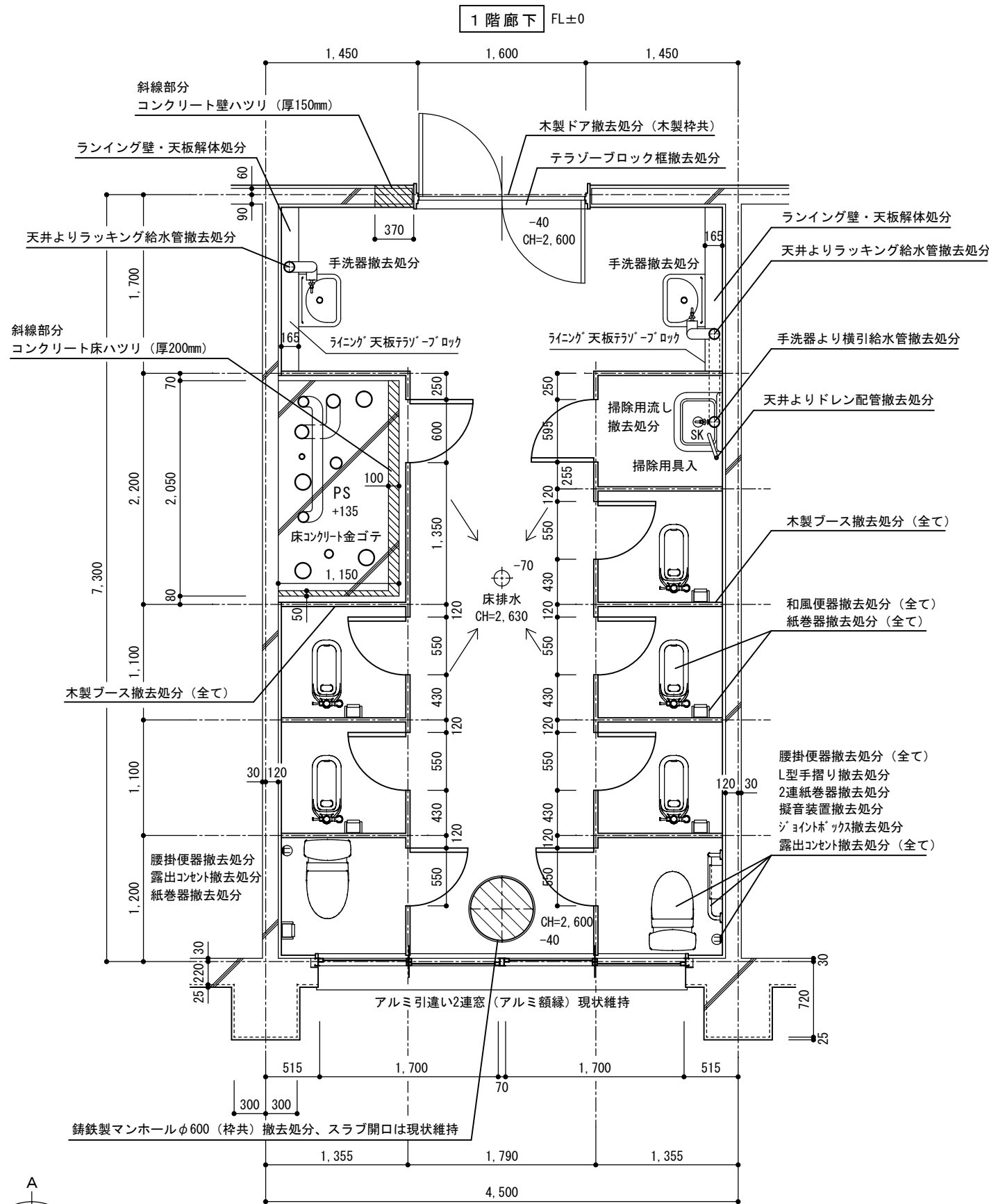
1階女子トイレ既存平面詳細図
