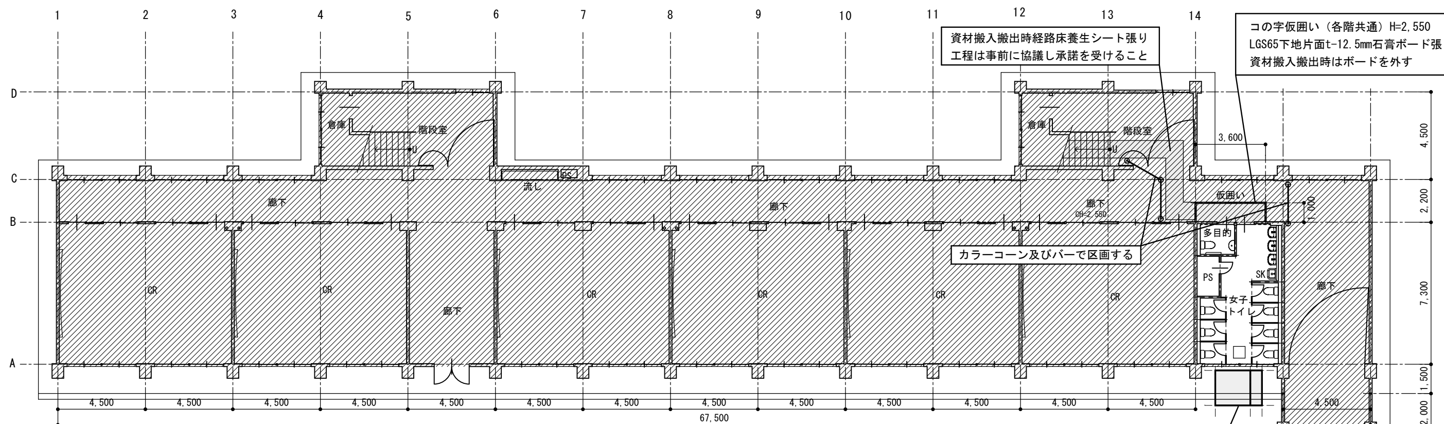
改修後1階平面図 1/200
