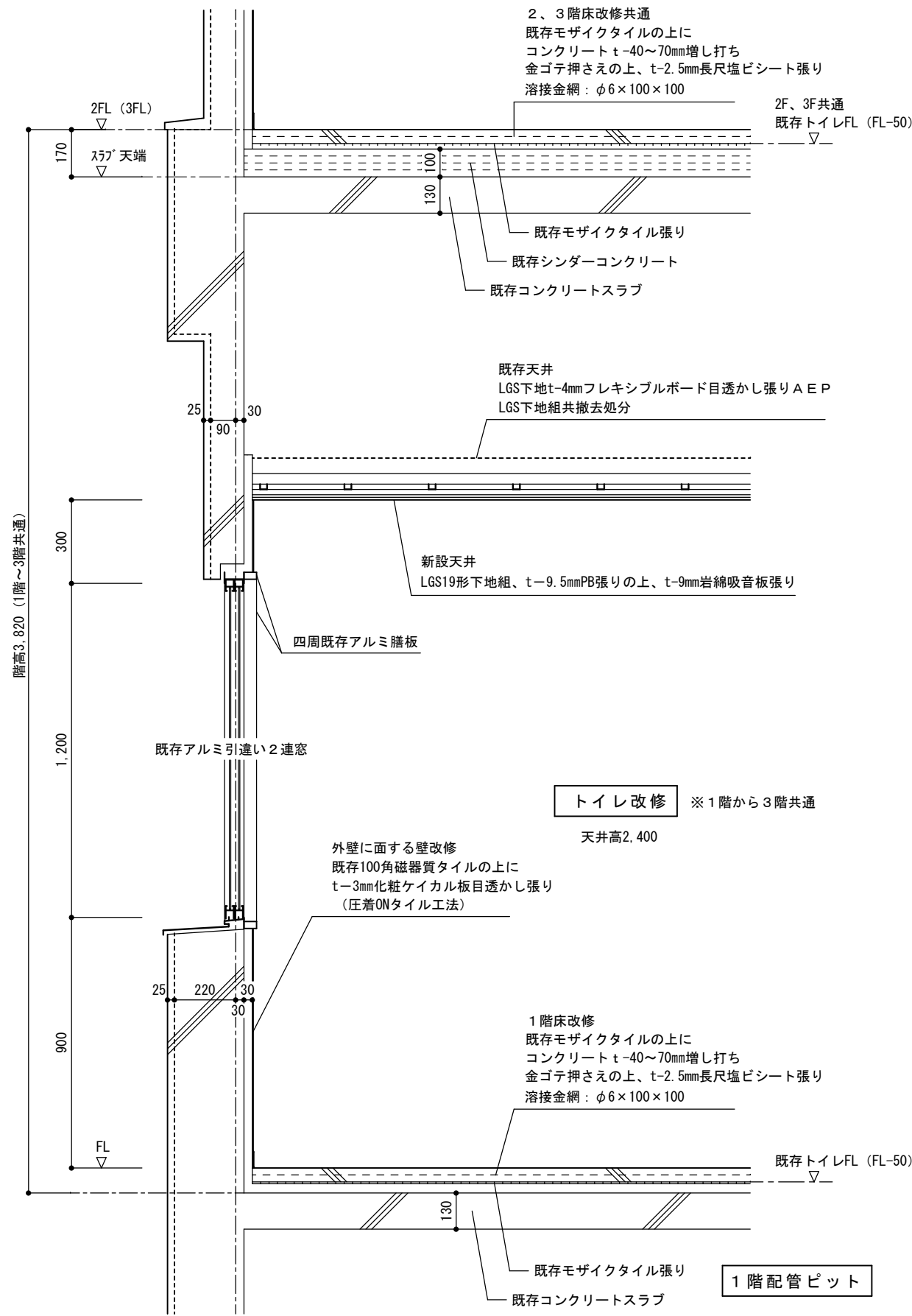
改修断面詳細図 1/20
