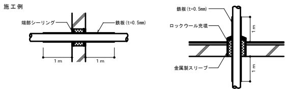
防火区画貫通部の処理
