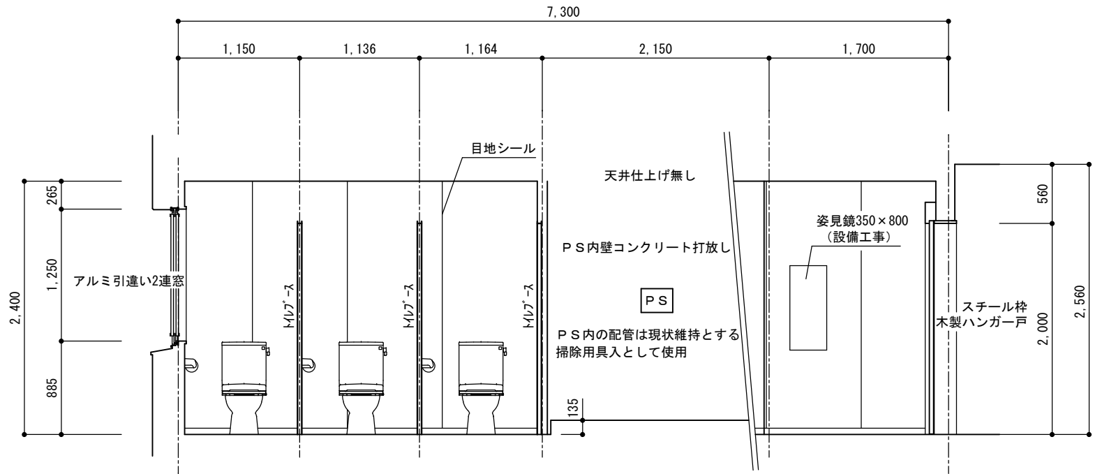
女子トイレ D面
