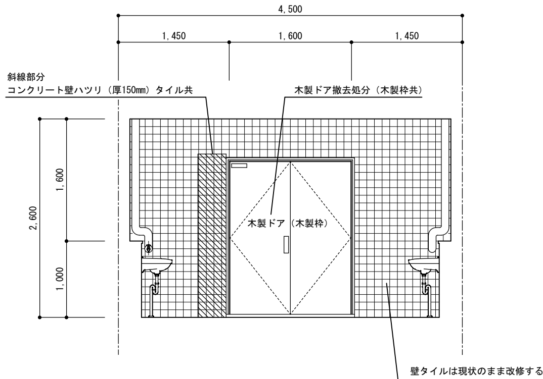
女子トイレ A面
