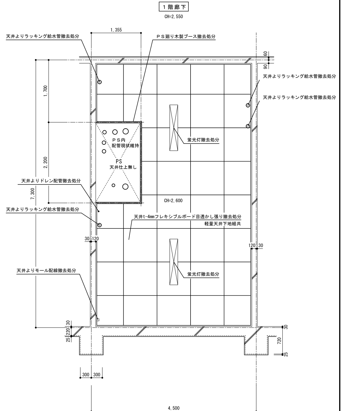
2階男子トイレ既存天井伏図
