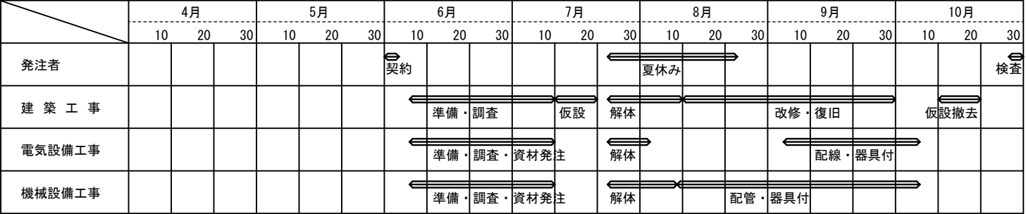
概略工程表 【参考】
