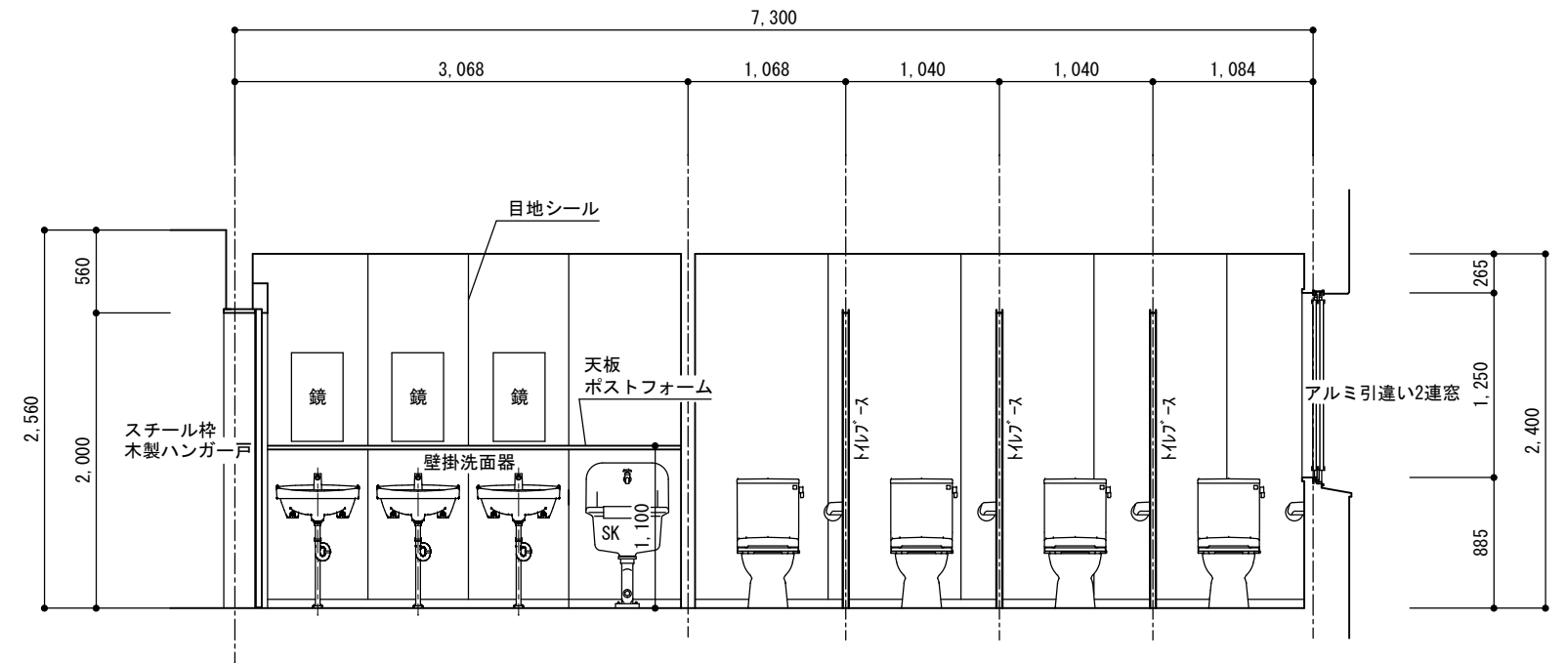
女子トイレ B面
