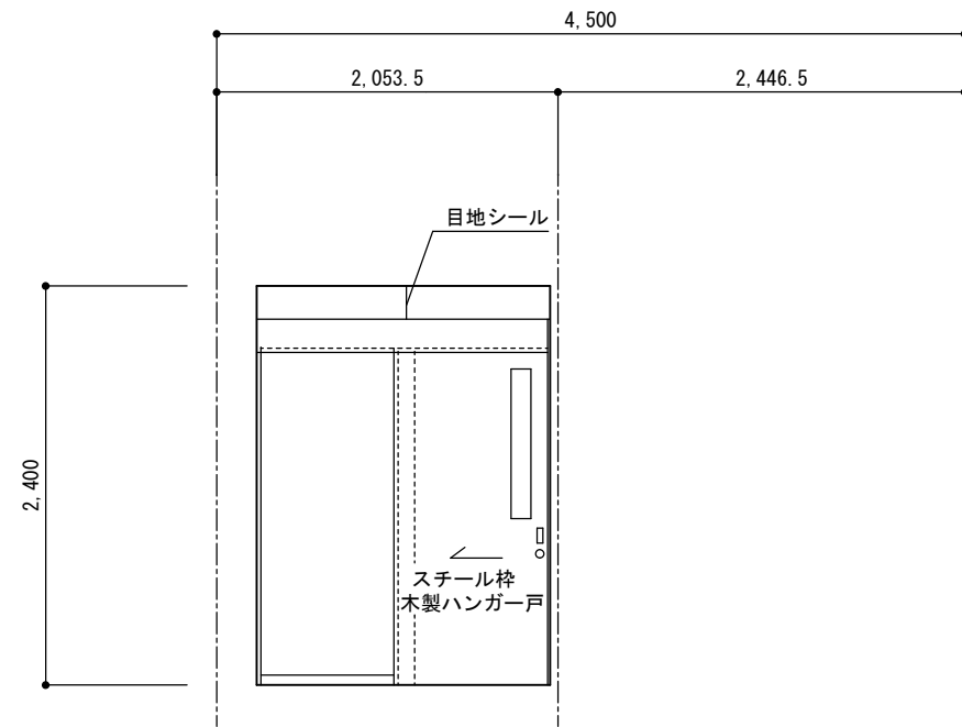
多目的トイレ A面
