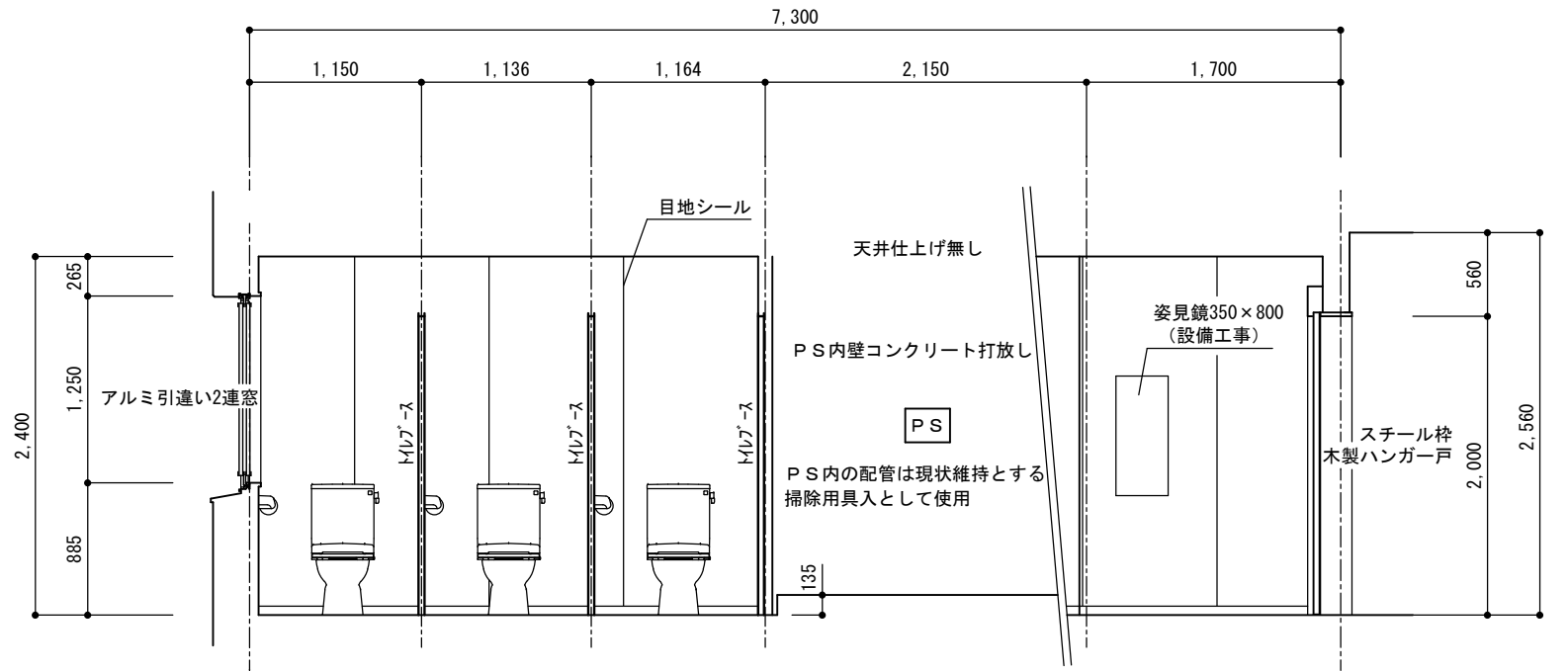
男子トイレ D面
