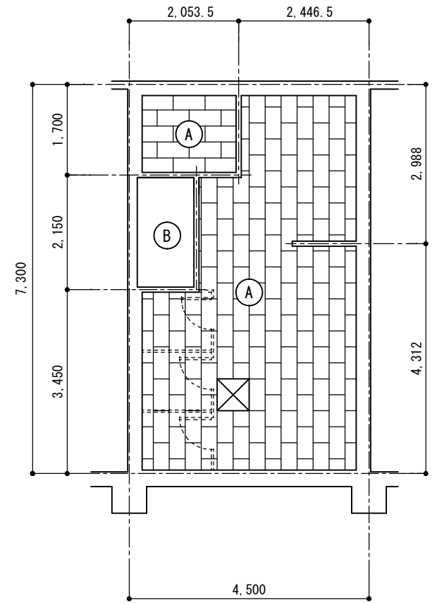
2階天井伏図 1/100
